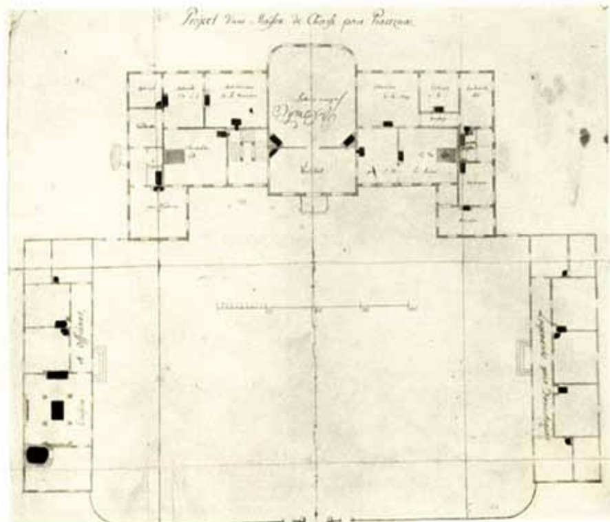
49 Projekt II. Schloß und Hofflagel. Erdgeschoß. C. F. Pöppelmann
